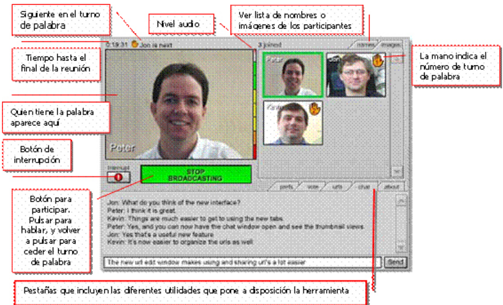
Figura 1. La aplicación FlashMeeting™ con algunas de sus características clave
