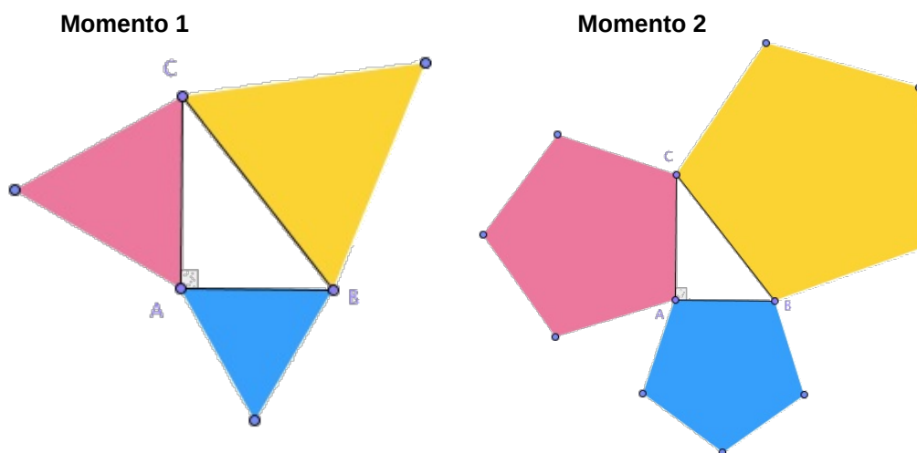
Figura 6: Prueba de Loomis.
