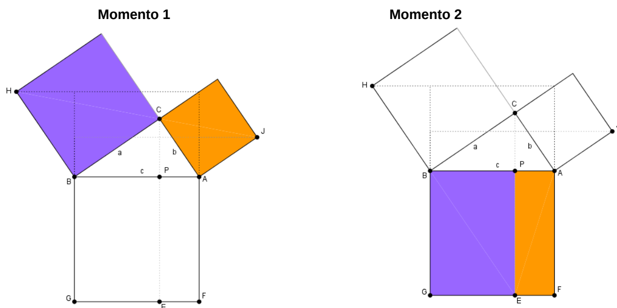
Figura 3: Prueba de Euclides.
