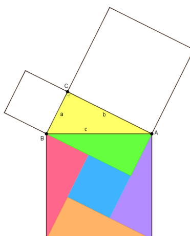
Figura 1: Cateto mayor/cateto menor = 2.
