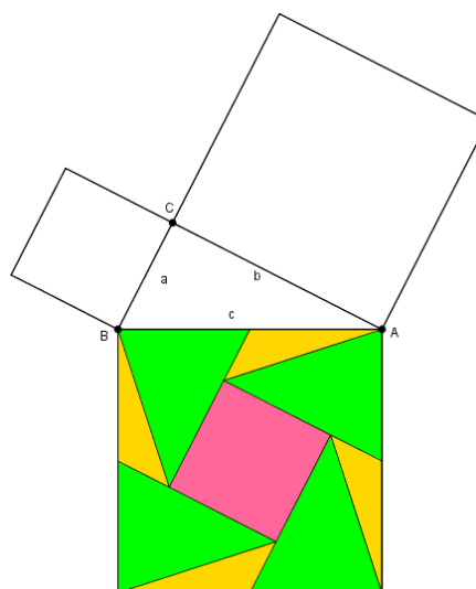
Figura 4: Prueba de Poo-Sung Park.
