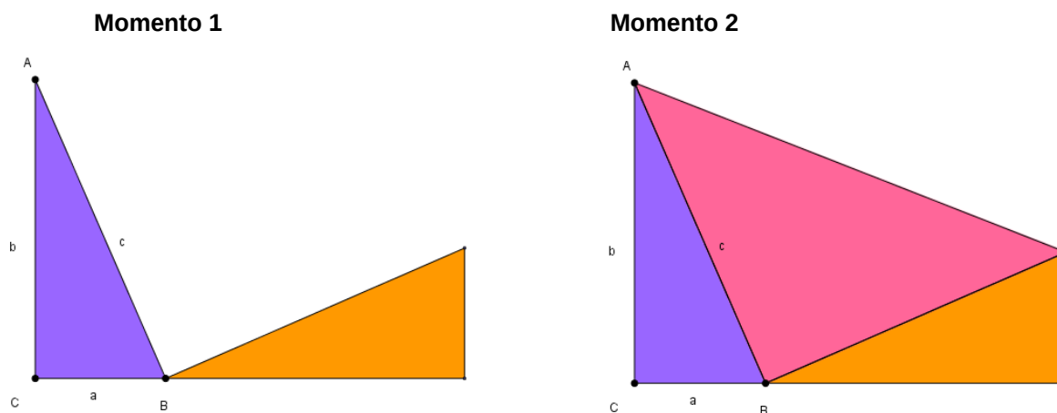
Figura 5: Prueba de Garfield.
