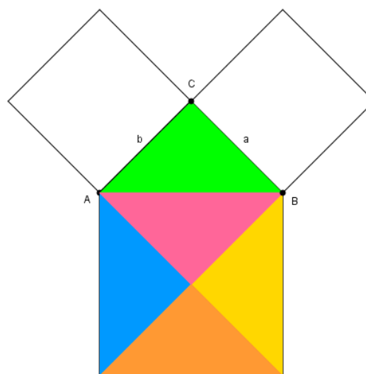
Figura 2: Prueba de Platón
