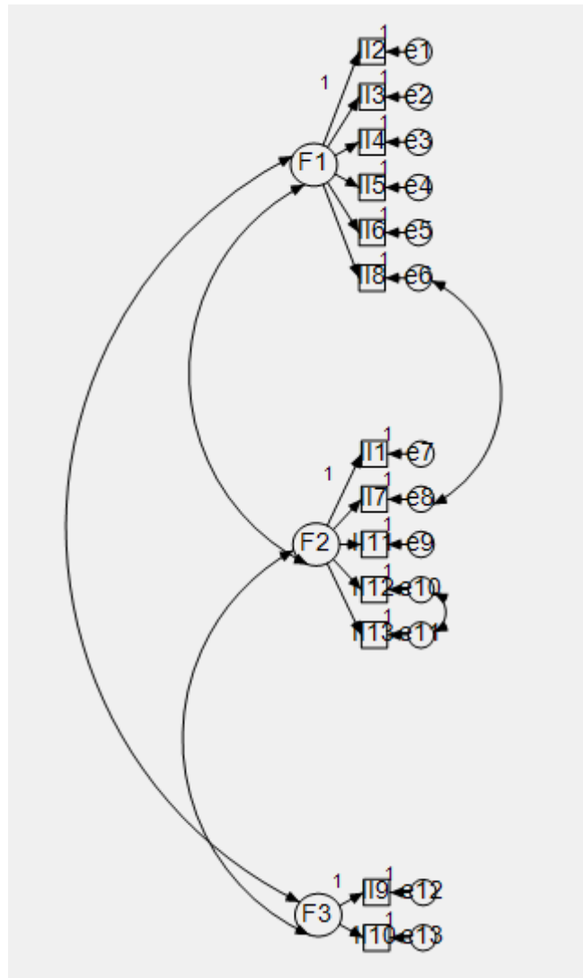
Figura 1. Modelo de 3 factores corregido
