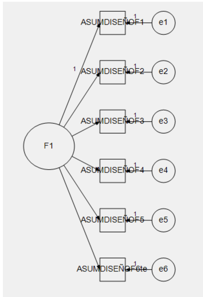
Figura 3. Modelo original de 6 subfactores
