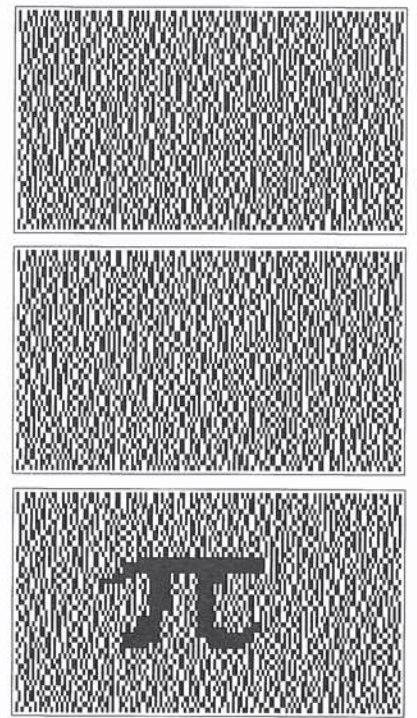
Figura 13. Símbolo \pi
