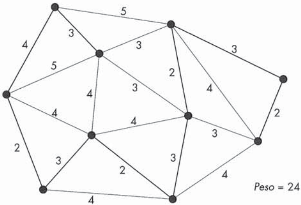
Figura 4. Diferentes aproximaciones a la solución óptima
